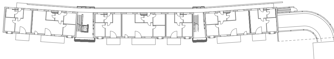
ERDGESCHOSS
