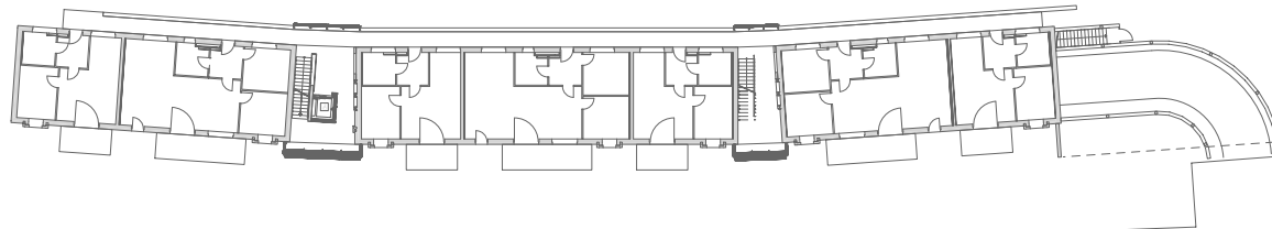
ERDGESCHOSS
